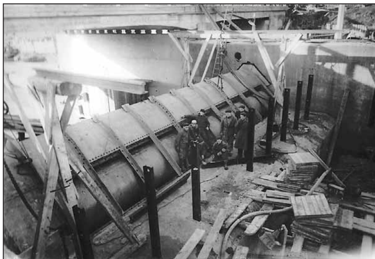
MONTÁŽ vlastního těla jezu s hydrostatickou automatizací.
