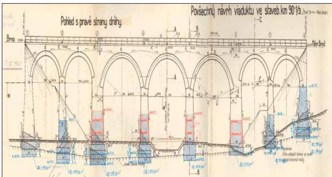
NÁVRH viaduktu na trati Brno – Nēm. Brod, úsek č. 8, jak byl schválen ministerstvem dopravy dne 21. 3. 1940.
