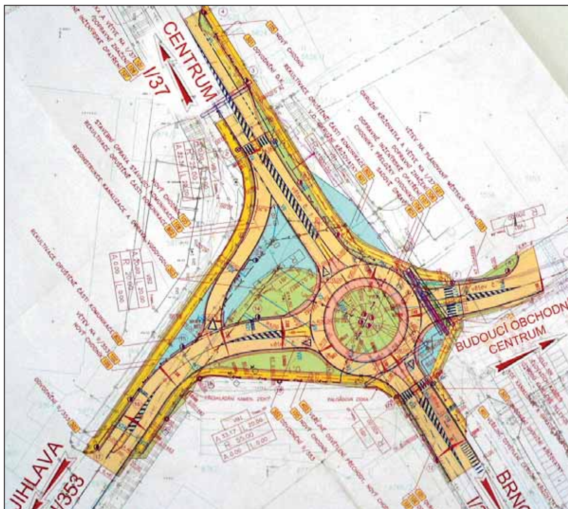
PROJEKT kruhové křižovatky u Enpeky, kterou staví firma SOVIS CZ, a.s. (Modře je naznačena předchozí křižovatka do T).
